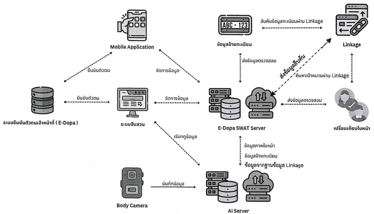
แผนภาพการส่งผ่านข้อมูลภายในระบบผ่านเว็บไซต์และแอปพลิเคชันบนโทรศัพท์เคลื่อนที่
