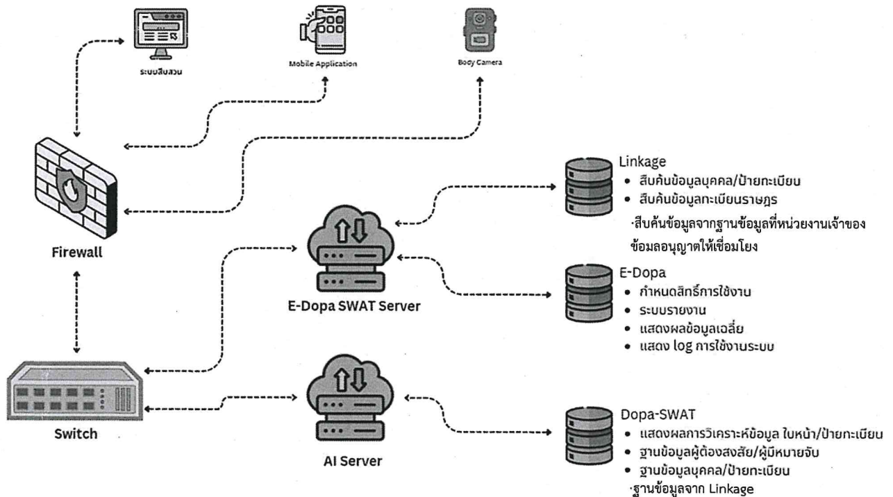
แผนภาพการเชื่อมโยงภายในระบบ
